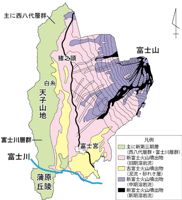
図 1-3 富士宮市の概略地質図 (津屋、1971・1986 を元に作成)
