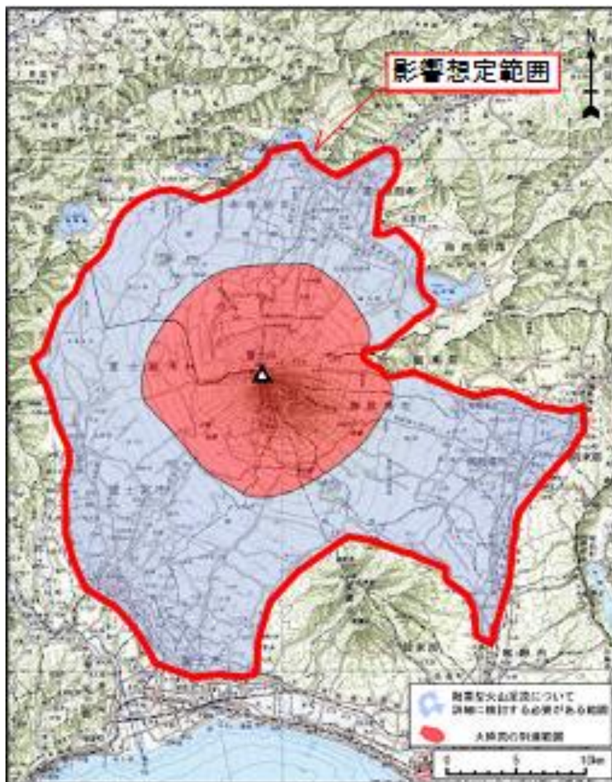
図4 融雪型火山泥流の影響想定範囲
