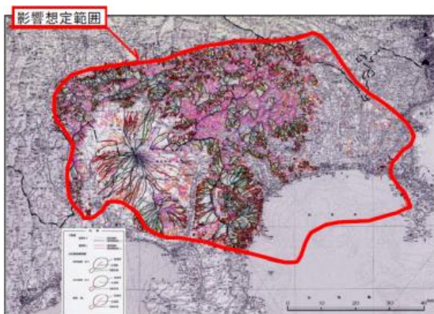
図5 降灰後土石流の影響想定範囲
