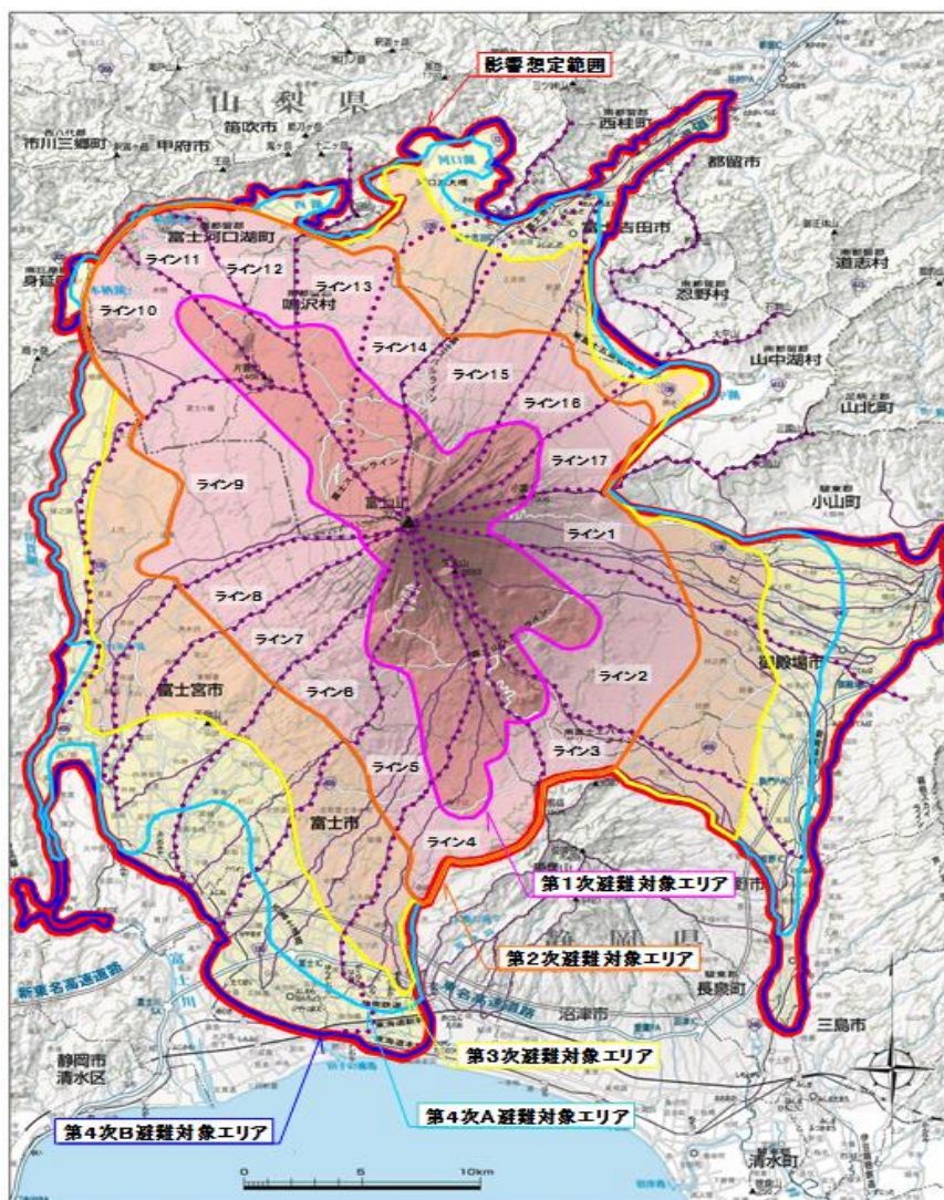
図1 想定火口範囲、噴石、火砕流・火砕サージ、溶岩流の影響想定範囲と避難対象エリア
